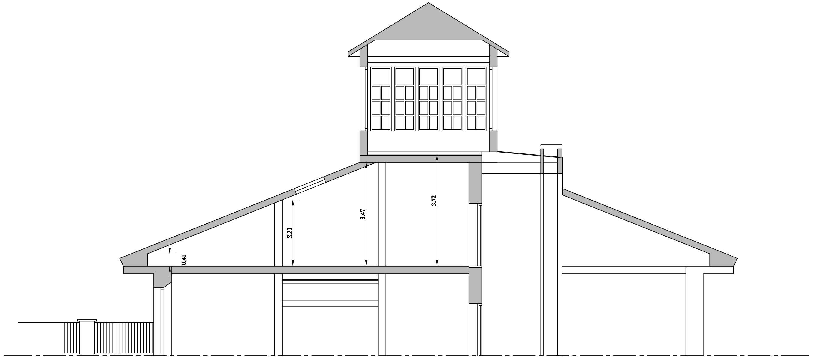
Sección A-B
